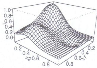
true function
